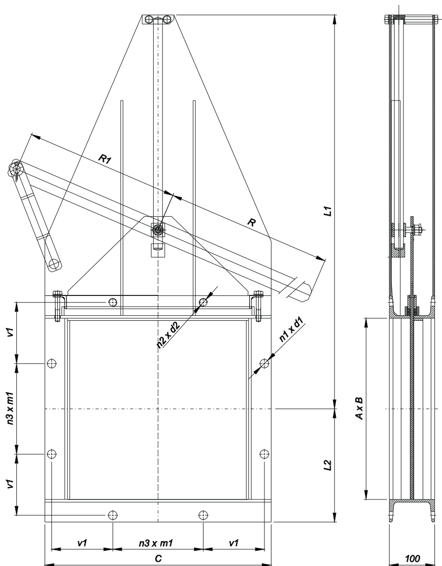
Obr.1 Základní rozměry
