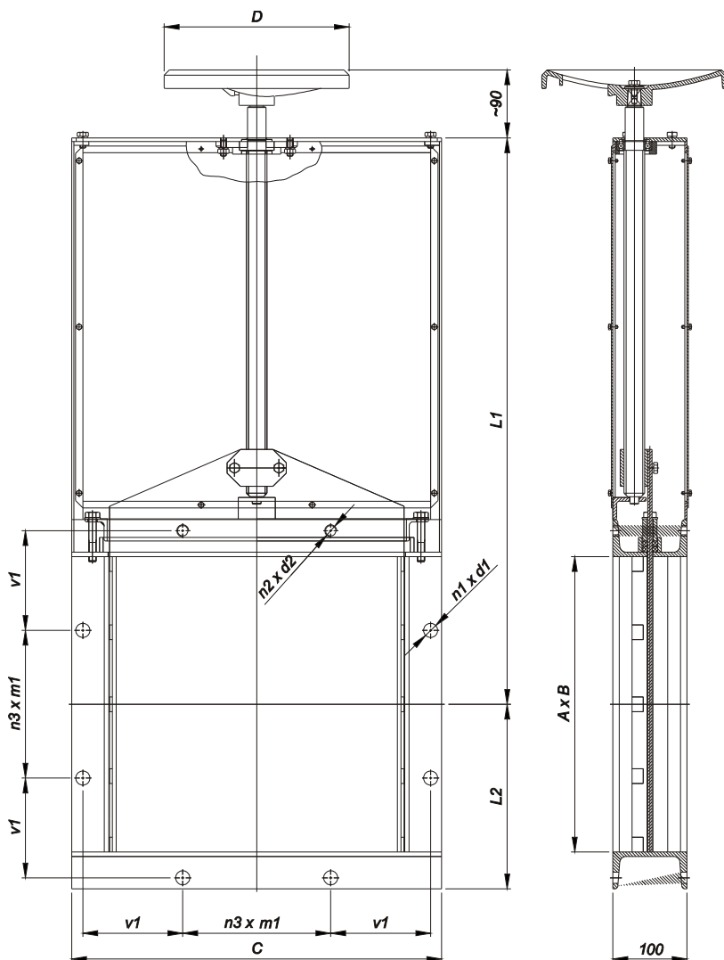
Obr.1 Základní rozměry
