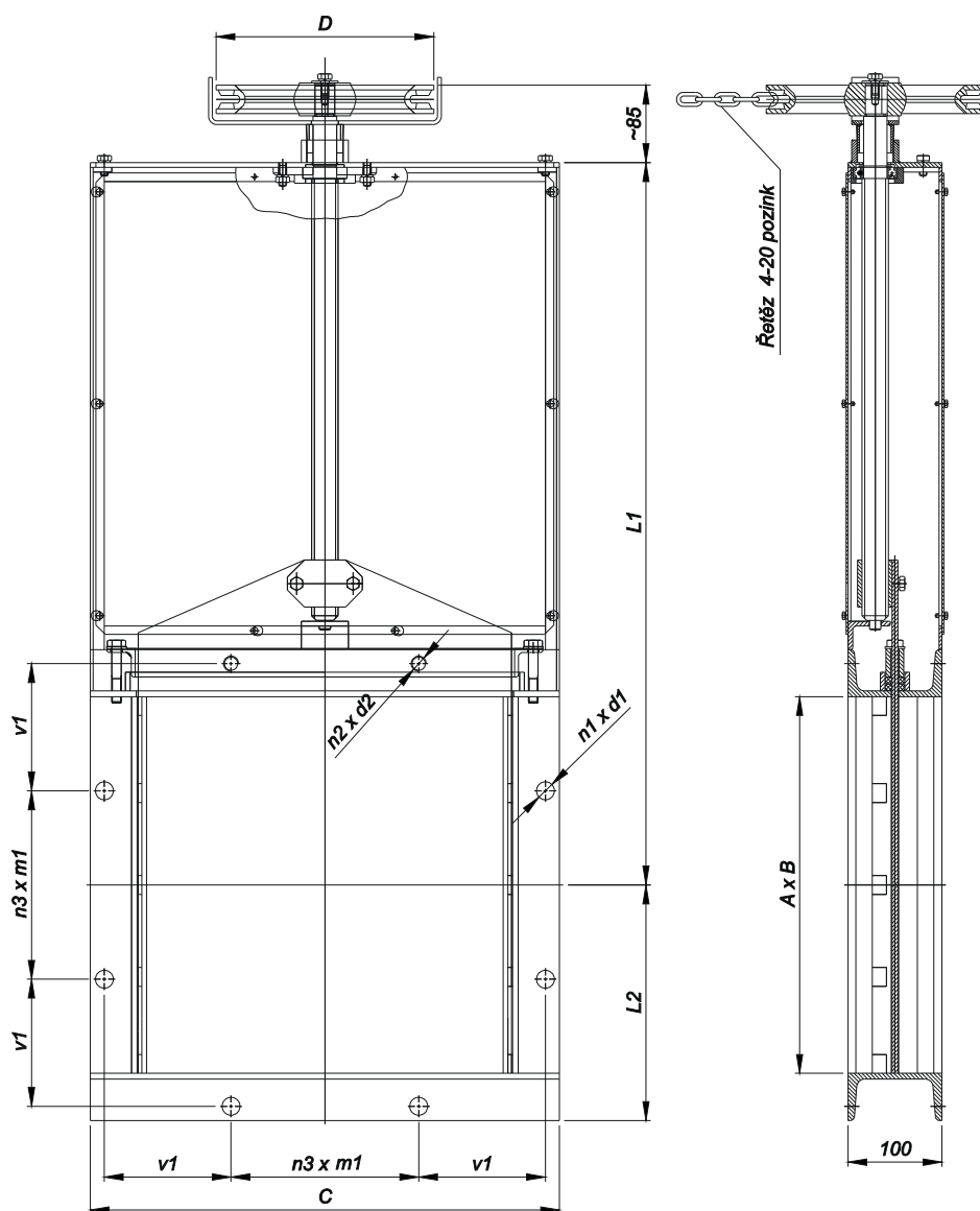
Obr.1 Základní rozměry
