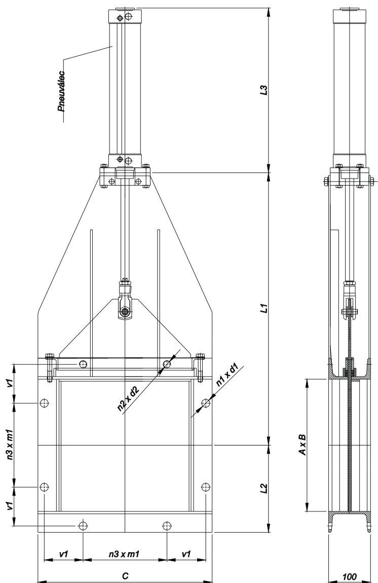
Obr.1 Základní rozměry
